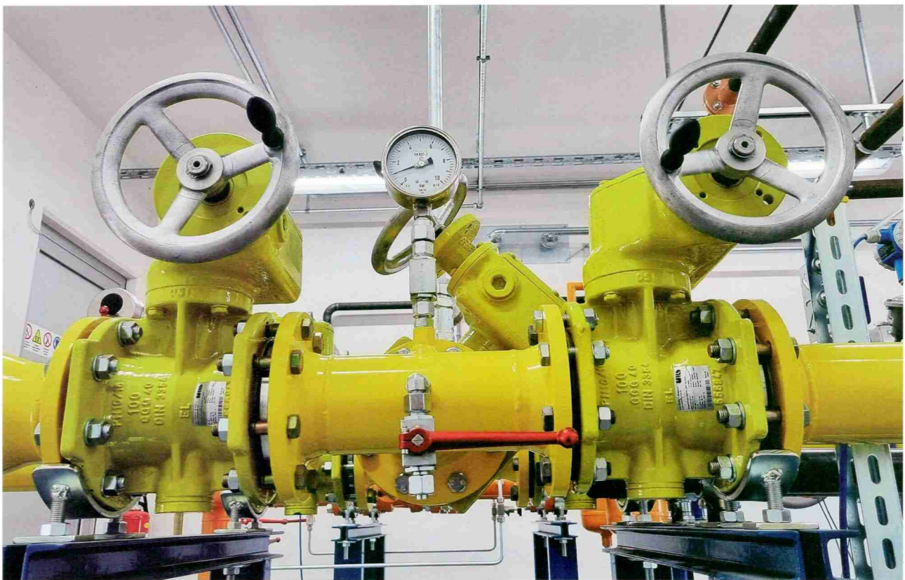
Les vannes papillon ont un émaillage bleu de protection totale à l'intérieur et un revêtement époxy jaune à l'extérieur. La commande des vannes se fait par un mécanisme à poussée dégressive avec volant.
